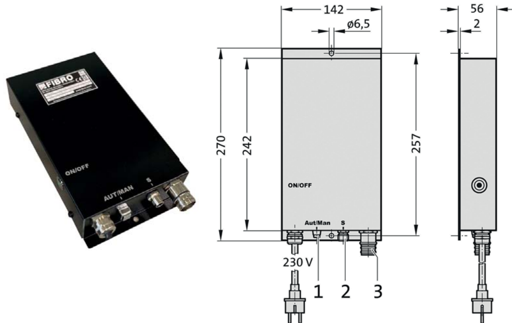
Abb. 3-2 Abmessungen Steuereinheit BLACK LINE
