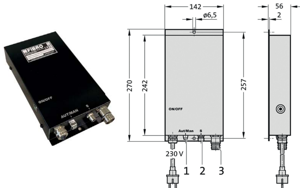
Rys. 3-2 Wymiary jednostki sterującej BLACK LINE
